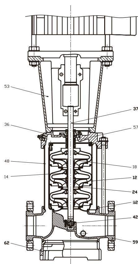
SBI(N)-32,45,64,90
